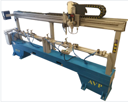
Spezielle Laserschweißmaschine
